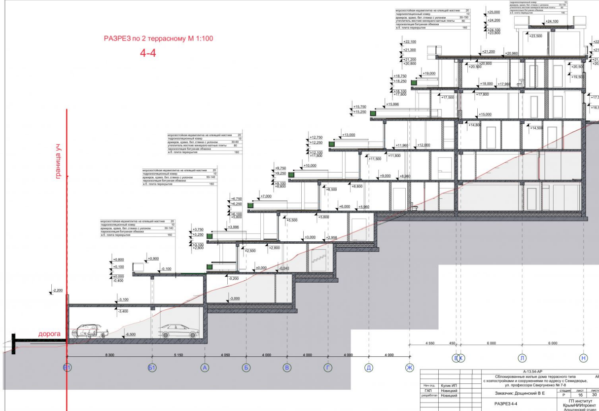
РАЗРЕЗ по внутреннему двору М 1:100
